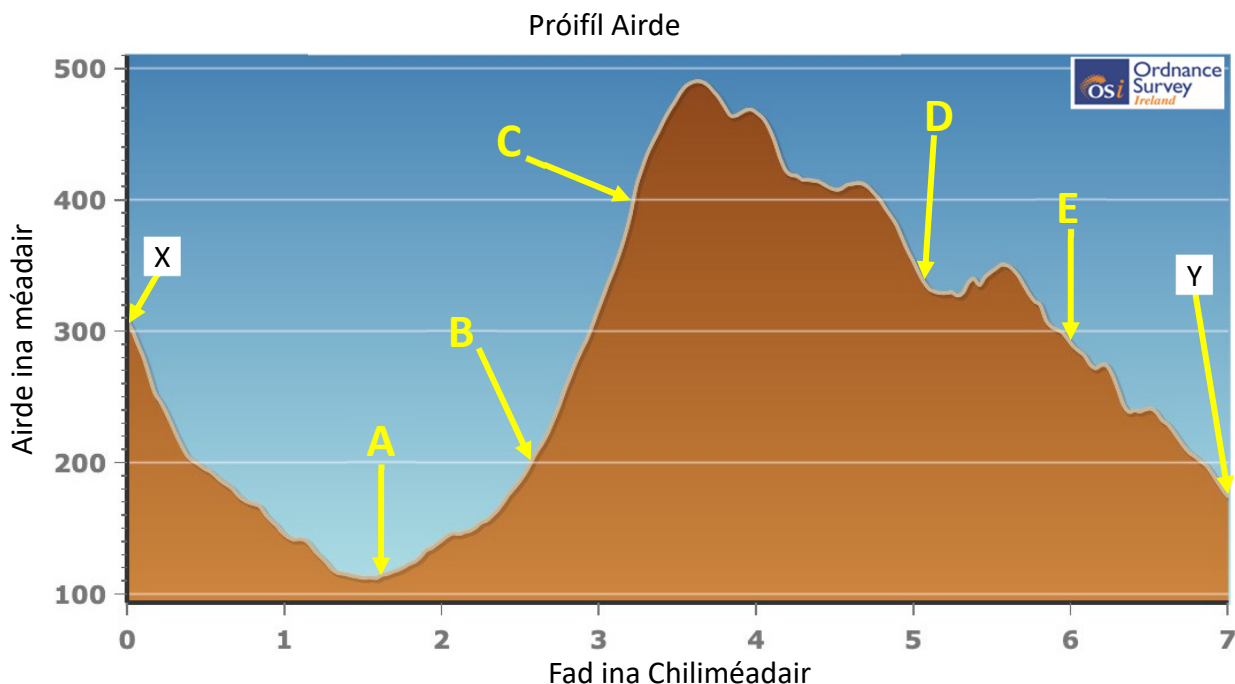
Fíor 1: Próifíl airde de thrasghearradh líne idir pointe X agus pointe Y .
